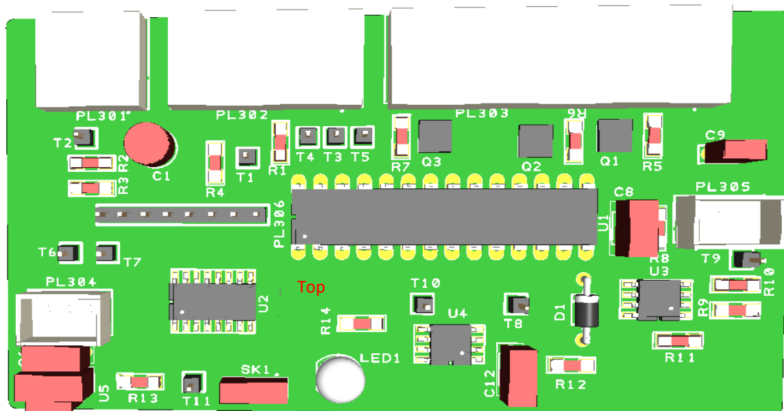
PCB3 MCU
