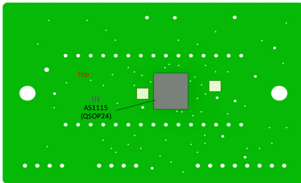
PCB1 CC-218 DISP
